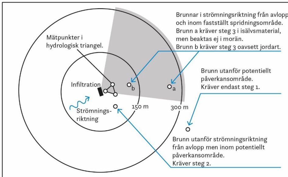
Figur 2. Principskiss över utredningsmodell med exempel på brunnspositioner. Figuren illustrerar gränser för potentiellt påverkansområde i morän (den lilla cirkeln) och isälvmaterial (den stora cirkeln) samt fastställt spridningsområde (det grå fältet). Vinkeln på det grå fältet kan variera. Med en flackare terräng och därmed svag gradient på grundvattnets lutning, blir spridningen bredare och spridningsriktningen mer oviss.
