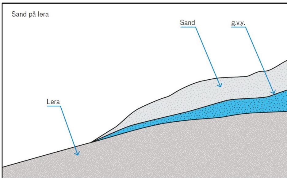
Figur 4. Planerar man att anlägga infiltrationen i ett jordlager med ett tätande lerlager (eller motsvarande) under, måste nedströms mäktighet på det jordlager som ska ta emot vattnet kontrolleras. G.v.y. är förkortning för grundvattenyta.
